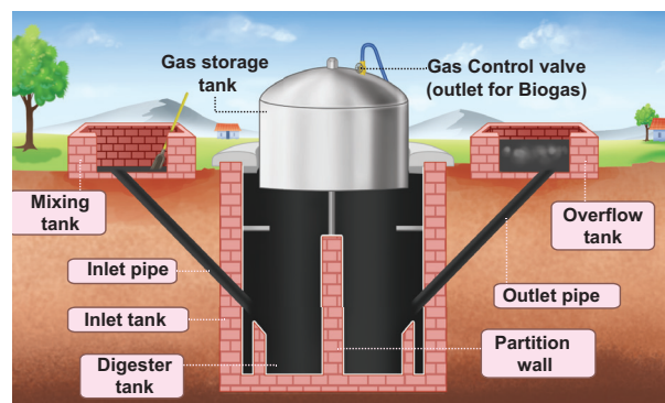
Fig. 8.3 Biogas Unit
